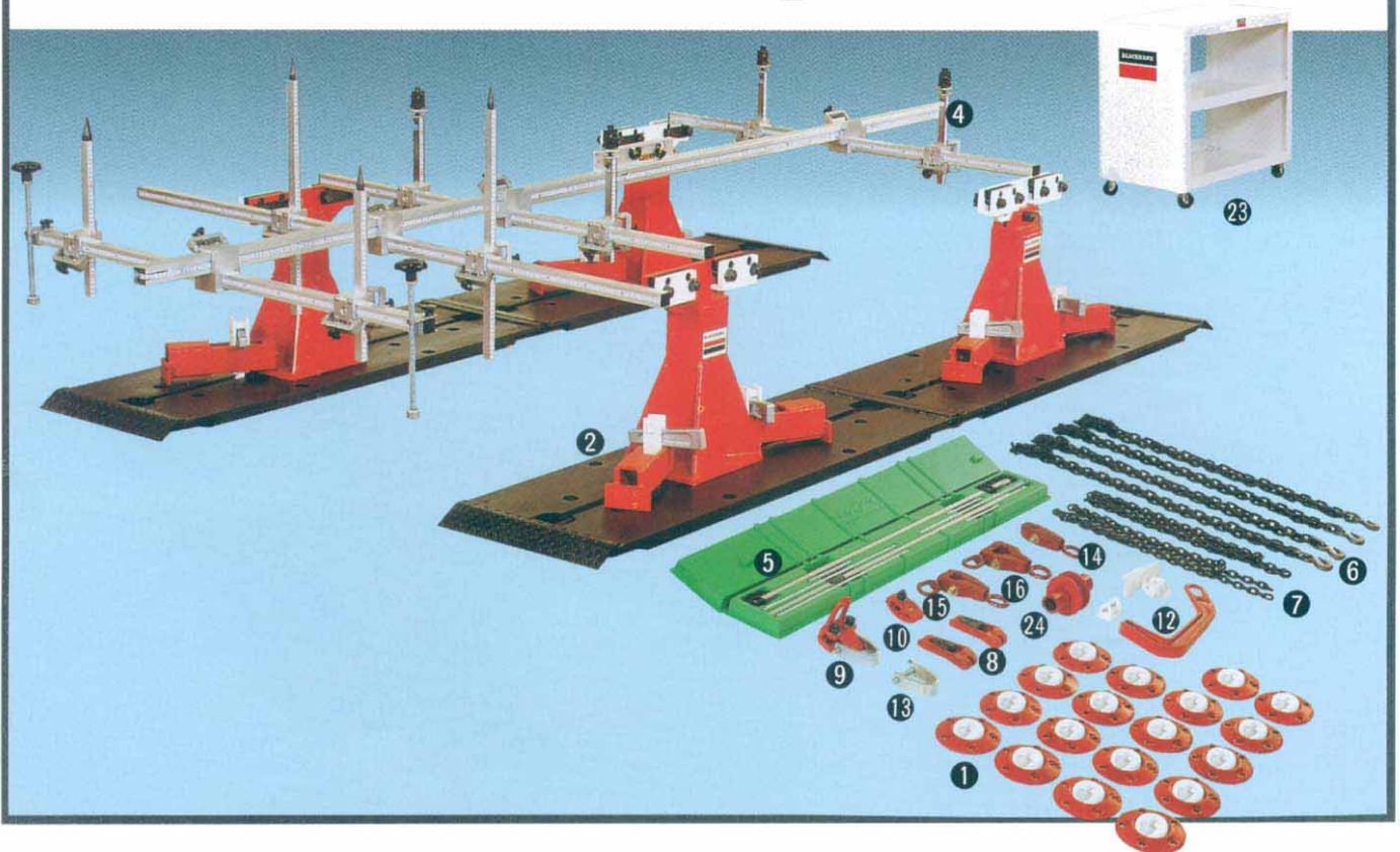
プリングポスト デラックスセット(アンカープレート式) PP-4400D
