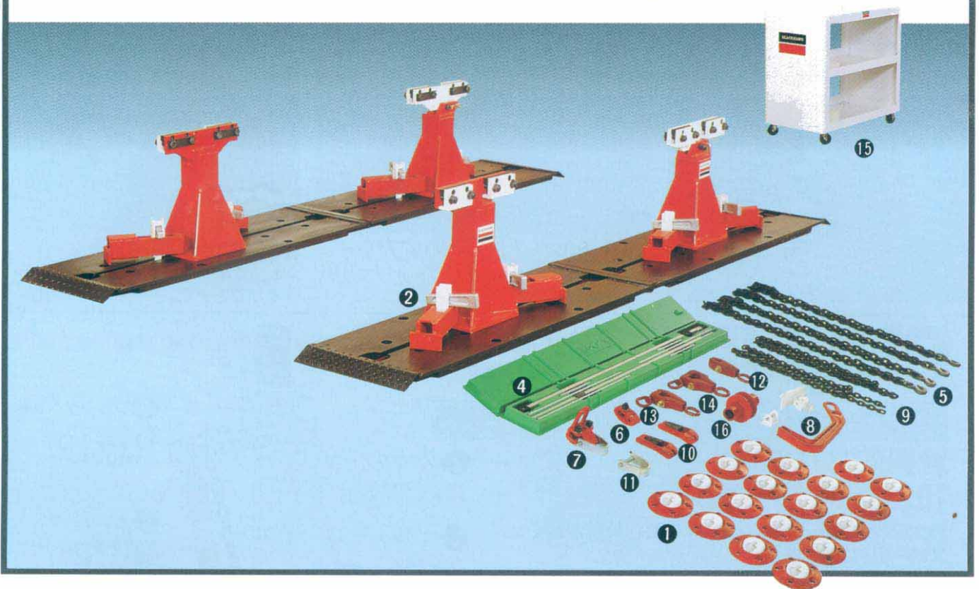
プリングポスト スタンダードセット(アンカープレート式) PP-4400S
