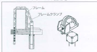
サスペンションリンクの固定(パーツ付)③
