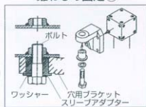
ロケットホールの固定⑥
