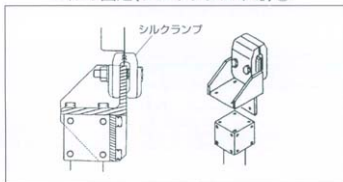
サスペンションリンクの固定(パーツ無し)④
