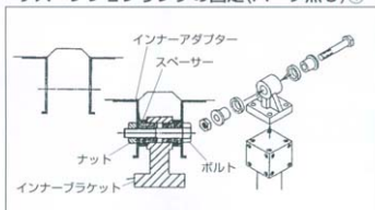
サスペンションリンクの固定(パーツ無し)④
